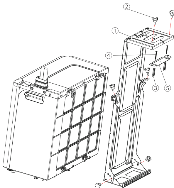
Composition du kit et mise en place sur l'unité extérieure
