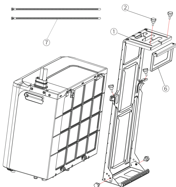
Composition du kit et mise en place sur l'unité extérieure
